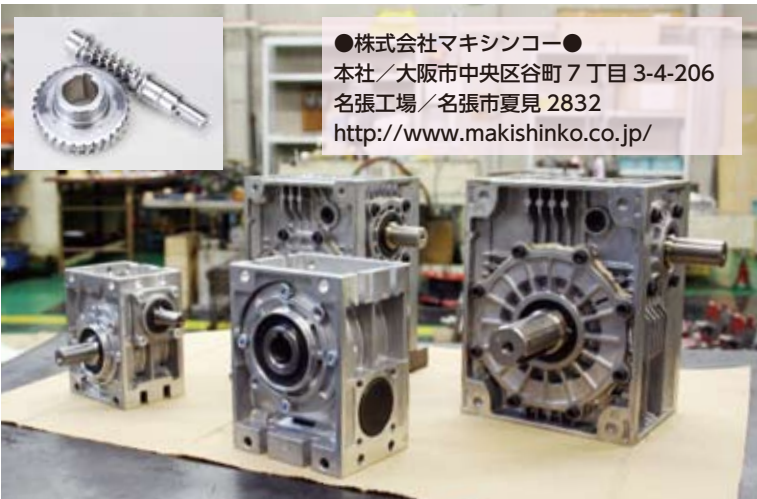
軽量化を進めるウォーム減速機。枠内は内部構造
